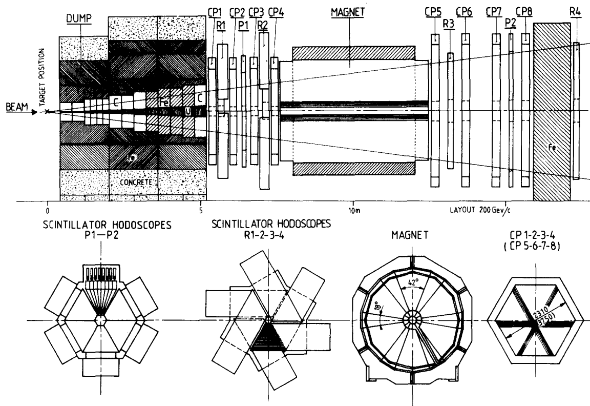
Fig. 1. NA 10 spectrometer.
